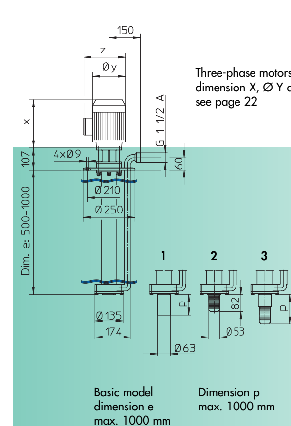
Dimensions F 706 PP-135
