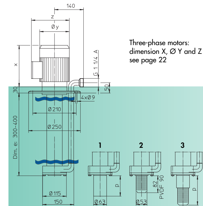
Dimensions F 716 PP1-115
