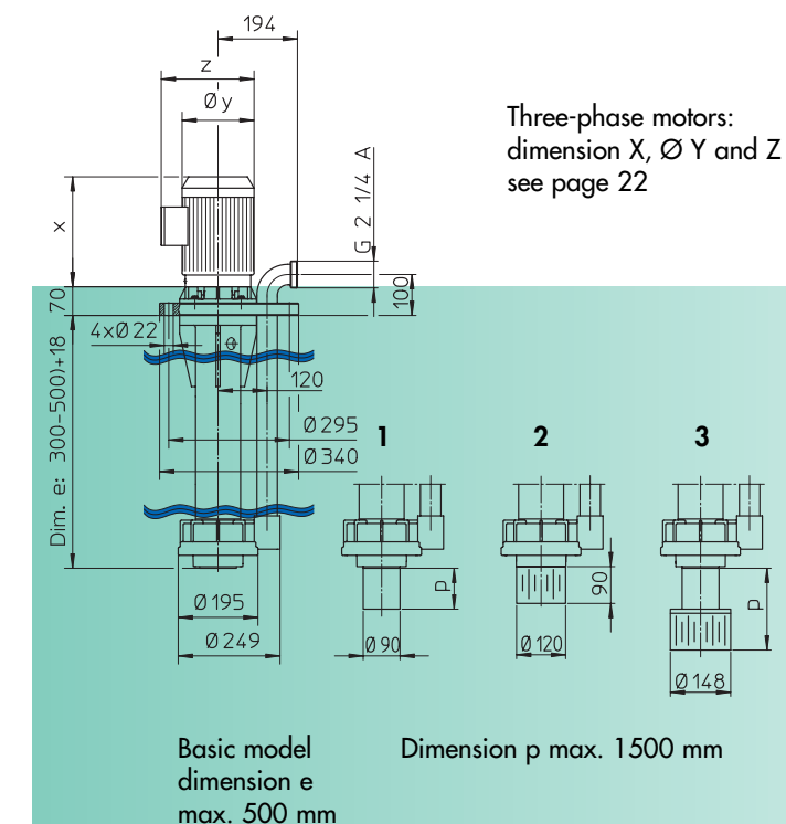
Dimensions F 716 PP1-185
